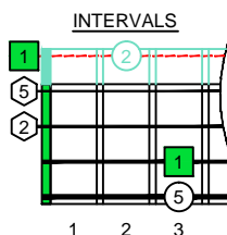
Csus2 arpeggio SEMITONOMETER
