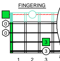
Csus2 arpeggio SEMITONOMETER
